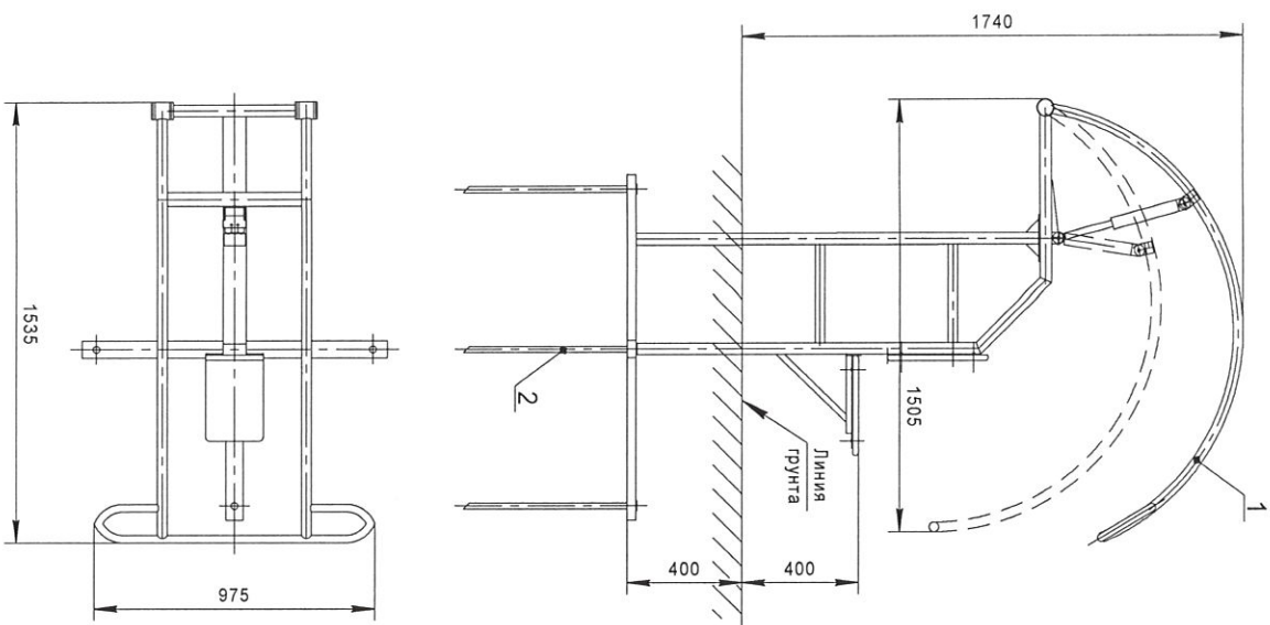
Рисунок 1 - Общие виды и установка изделия
